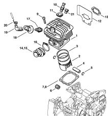
Válec
