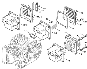
Tlumič výfuku
