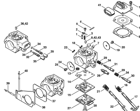
Karburátor HD-14, HD-16, HD-24
