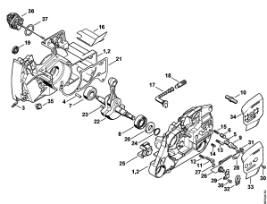
Kliková skříň, klikový hřídel
