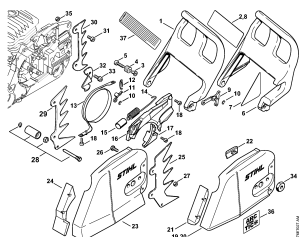
Řetězová brzda, víko řetězky
