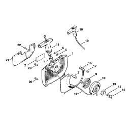
Startovací zařízení
