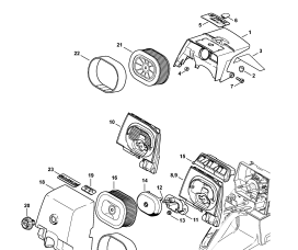
Kryt, vzduchový filtr
