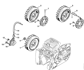
Zapalování
