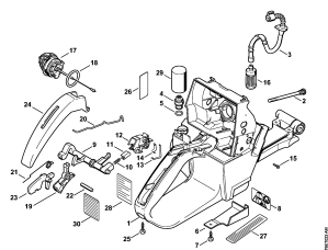
Těleso nádrže
